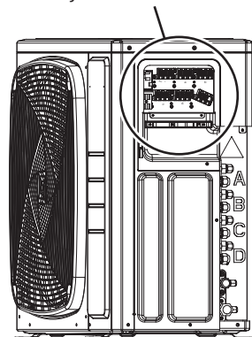
Terminal y Área del Cableado
