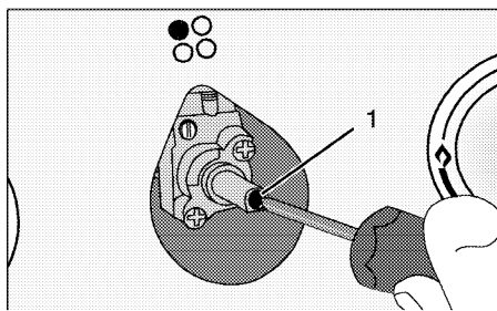
1. Vis de réglage du débit de gaz
