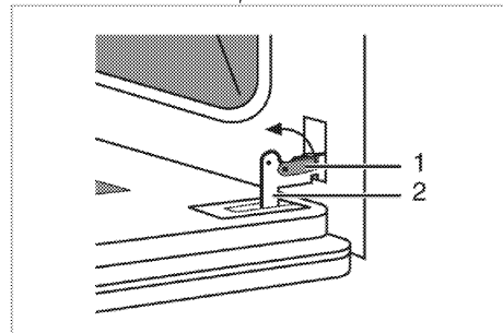
1 Charnière de serrage 2 Charnière
