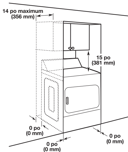
Vue d'avant, encastrement
