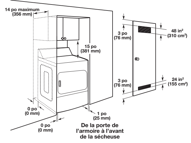
Vue latérale, encastrement dans une armoire
