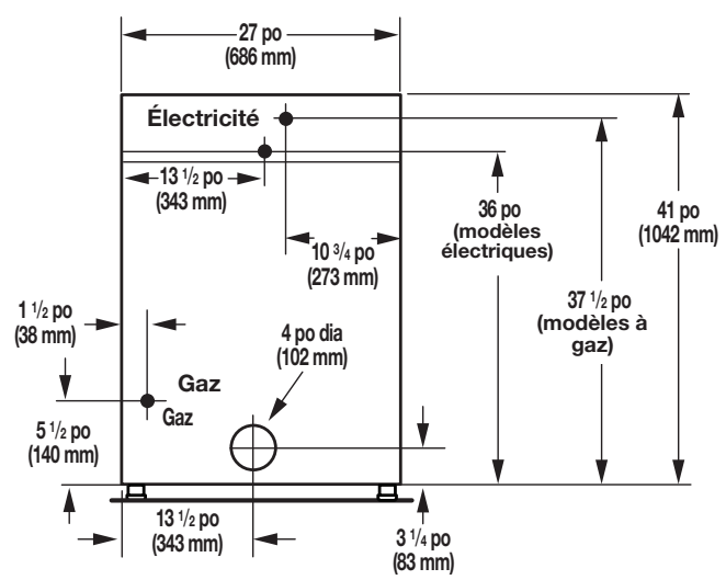
Vue arrière
