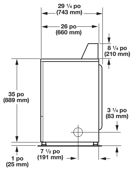
Vue latérale
