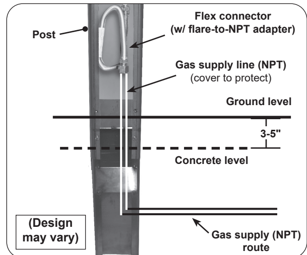
Fig. 28-3 Pour concrete & install post
