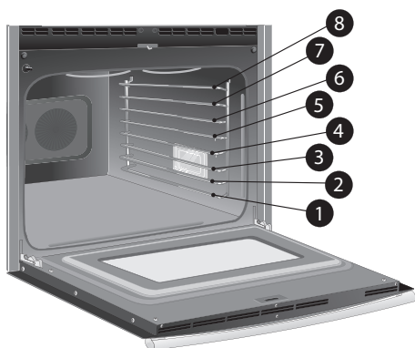
Figure 18 : Emplacement des grilles
