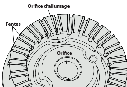
Figure 26 : Composants de brûleurs scellés
