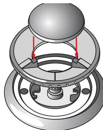
Figure 28 : Positionnement d'un capuchon de brûleur
