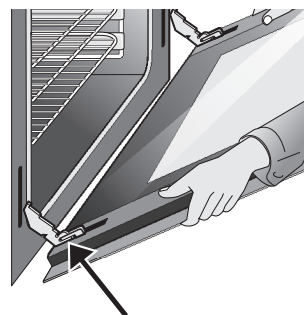
Figure 39 : Dépose du balconnet de porte
