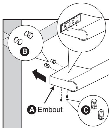
Assembler la poignée du congélateur
