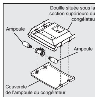
Lumière du congélateur
