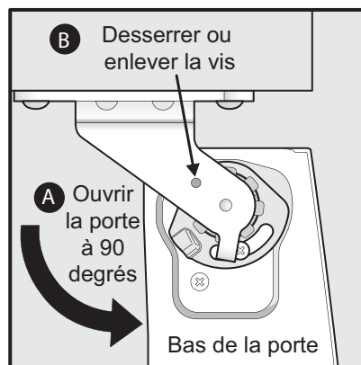
Desserer/Enlever la vis
