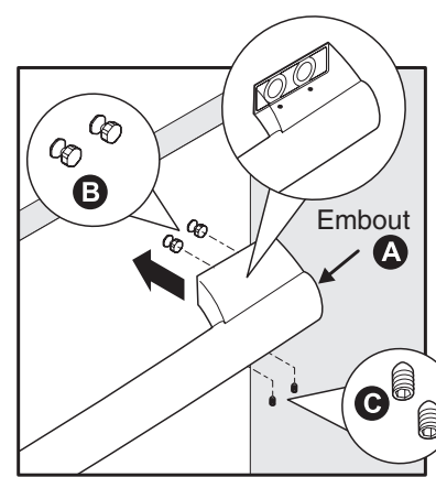
Assembler la poignée du congélateur
