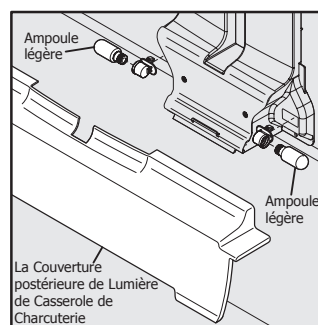
Lumière dans le mur arrière
