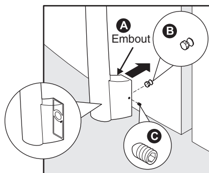
Assembler les poignées du réfrigérateur
