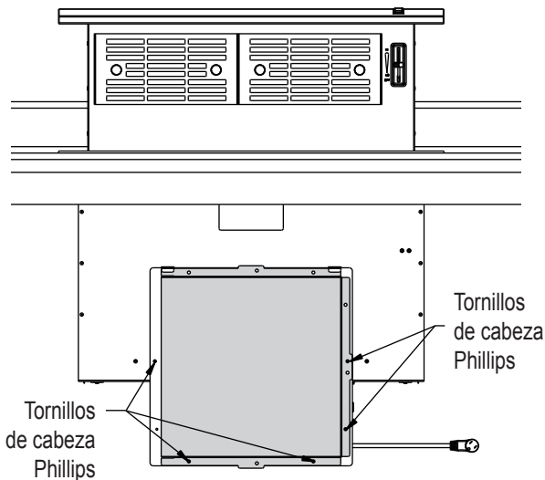
Figura 2: descarga izquierda
