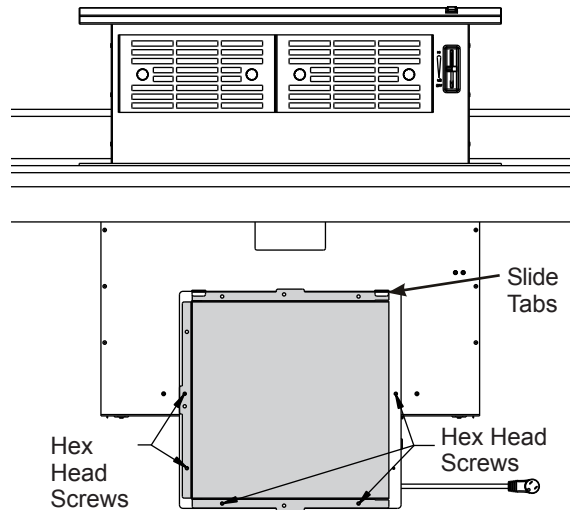
Fig. 3 - Discharge right
