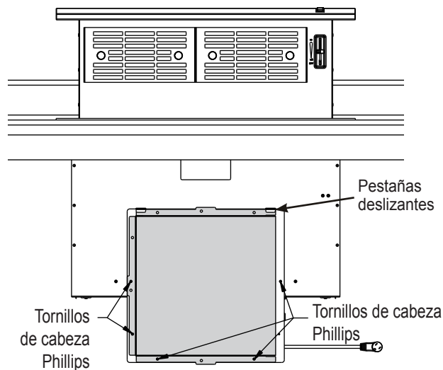
Figura 3: descarga derecha
