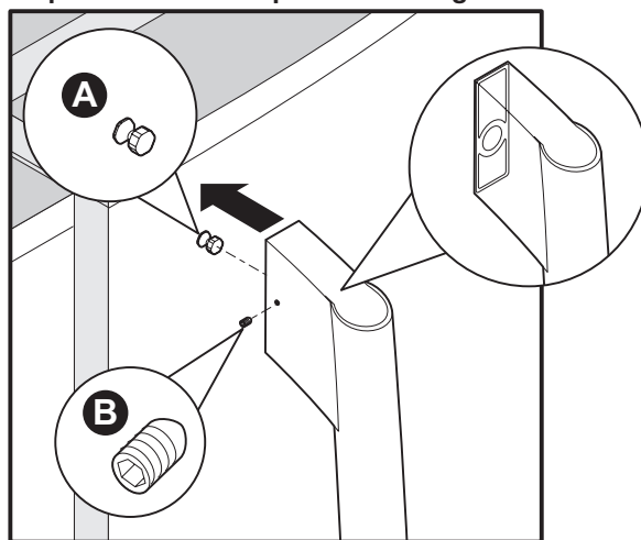
Tapa del extremo superior del refrigerador
