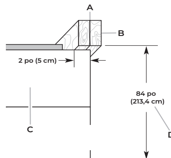
A. Deux panneaux de 2 po x 4 po x 32 po (5 cm x 10 cm x 81 cm) B. Fixer aux montants avec six vis no 8 x 3 po (7,6 cm). C. Couvercle du compresseur D. Distance entre le bas du panneau antibasculement et le plancher
