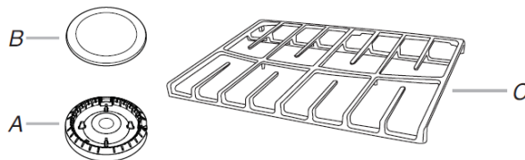
A. Base du brûleur B. Chapeau de brûleur C. Grille du brûleur (varie en fonction du modèle)
