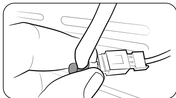
A. Fils couplés
