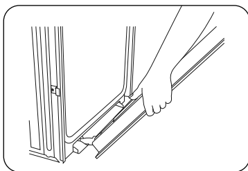
A. Ranura de la cavidad del horno para la traba de la bisagra de la puerta
