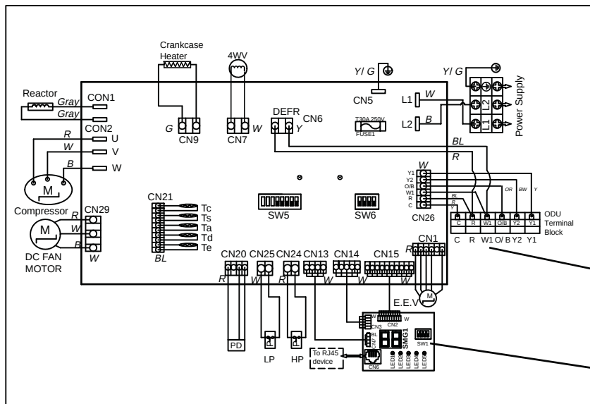
Figure 19. Schéma de câblage 18K/24K/30K/36K/42K/48K
