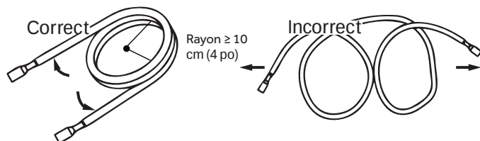
Figure 4. Rayon de courbure minimal
