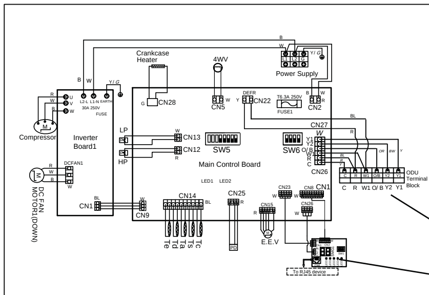
Figure 20. Schéma de câblage 60K
