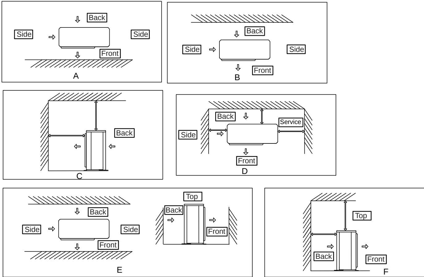
Figure 2. Configurations de dégagement pour une seule unité
