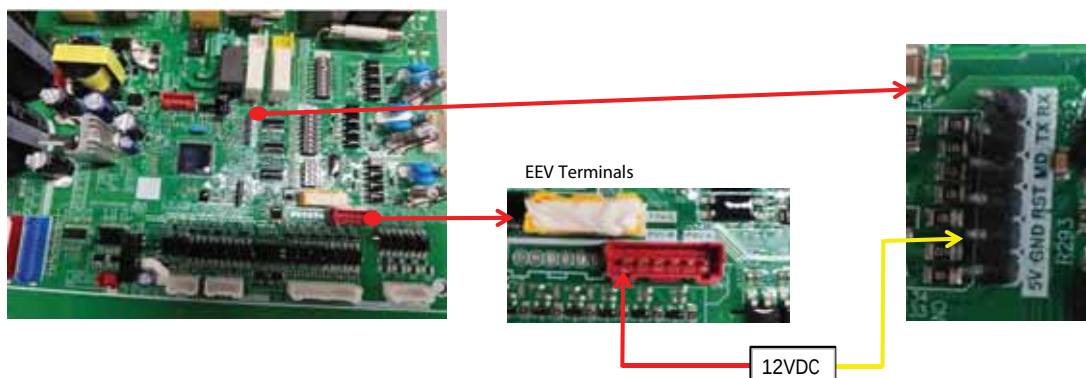
30K & 36K & 42K & 48K & 60K EEV(6-pin, 6 wire)
