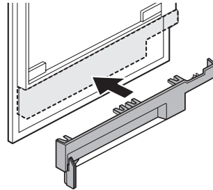
Freezer/FreshZone+ Door
