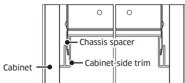
Cabinet Depth : 25"
