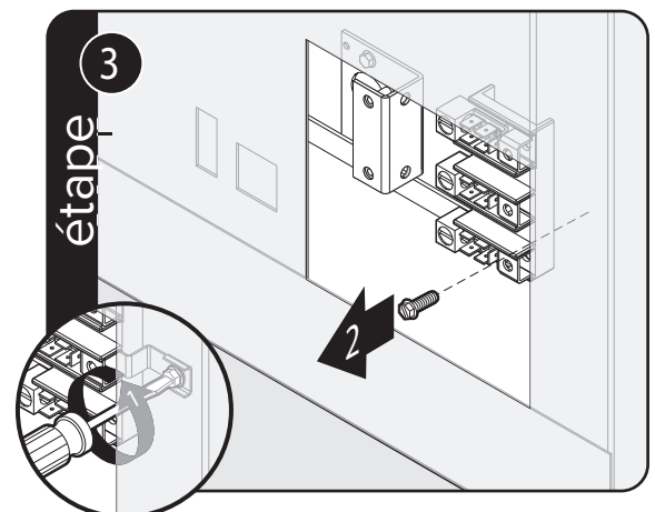
Retirez la vis de mise à la terre. Coupez et mettez au rebut la courroie de masse.
