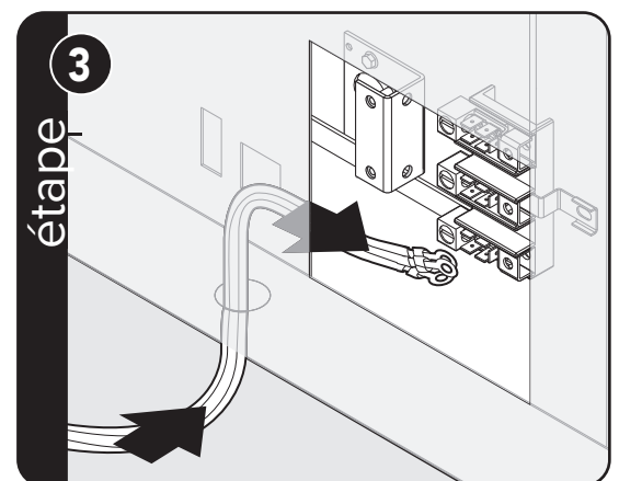
Faites passer le cordon d'alimentation par le trou situé en bas du dos de la cuisinière.
