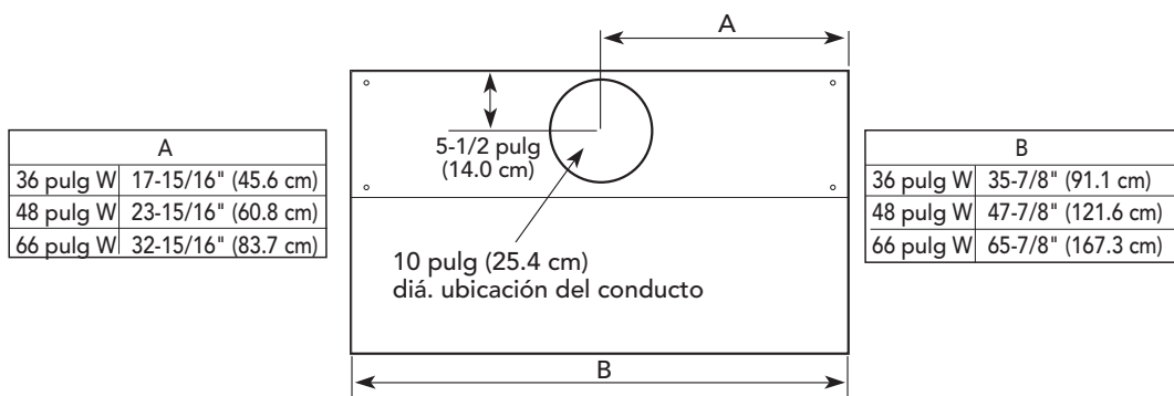
Vista superior
