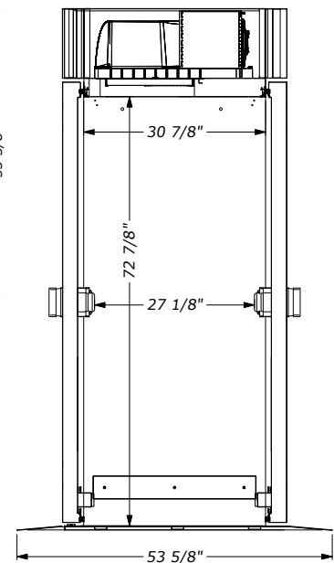
Back UCRE733/766
