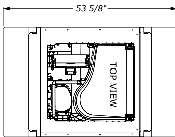
Top UCRE733
