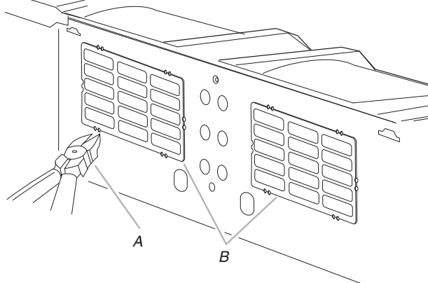
A. Alicate cortaalambres diagonal B. Cubierta de ventilación rectangular
