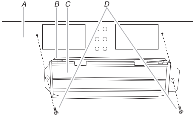
A. Parte posterior del horno de microondas B. Ensamblaje de la compuerta de tiro C. Hoja de la compuerta de tiro D. Tornillos para metal laminado #6 x 3/8" (2)
